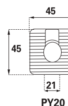
Dettaglio del supporto per piastra PICC2B Support detail for PICC2B plate
