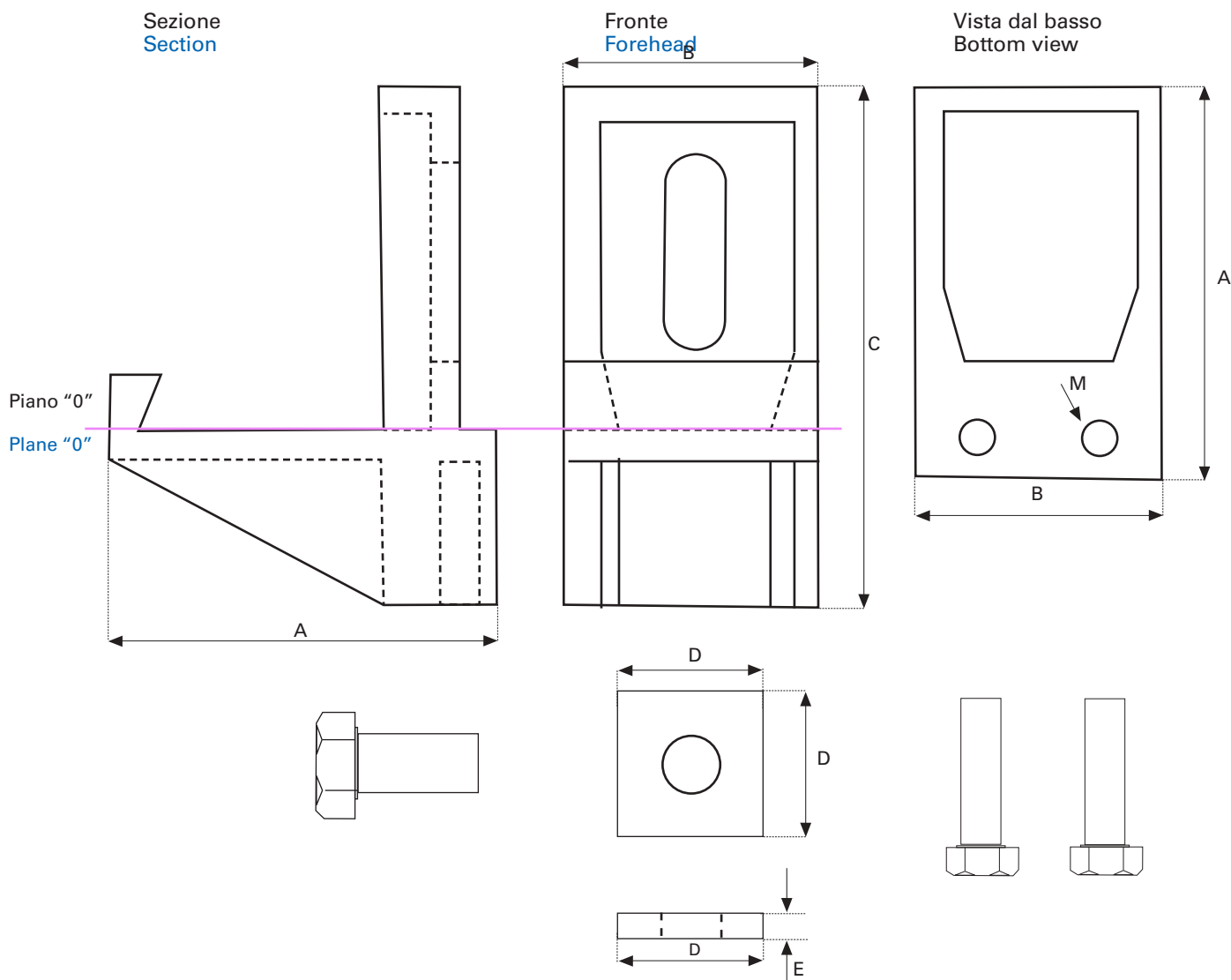
Mensola - Bracket
